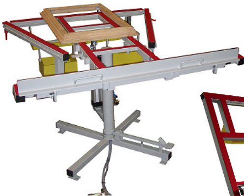
Dreh- Kipptisch RU-4 ▲
